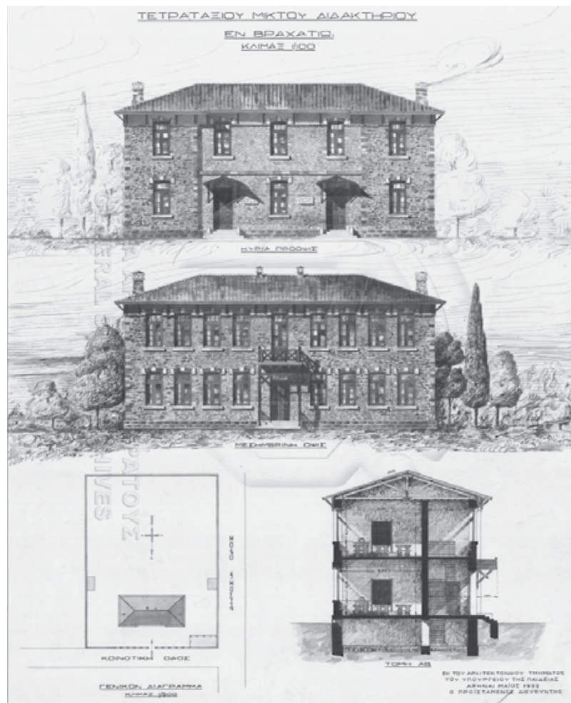
Μελέτη Διδακτηρίων Βραχατίου, έτους 1922.
